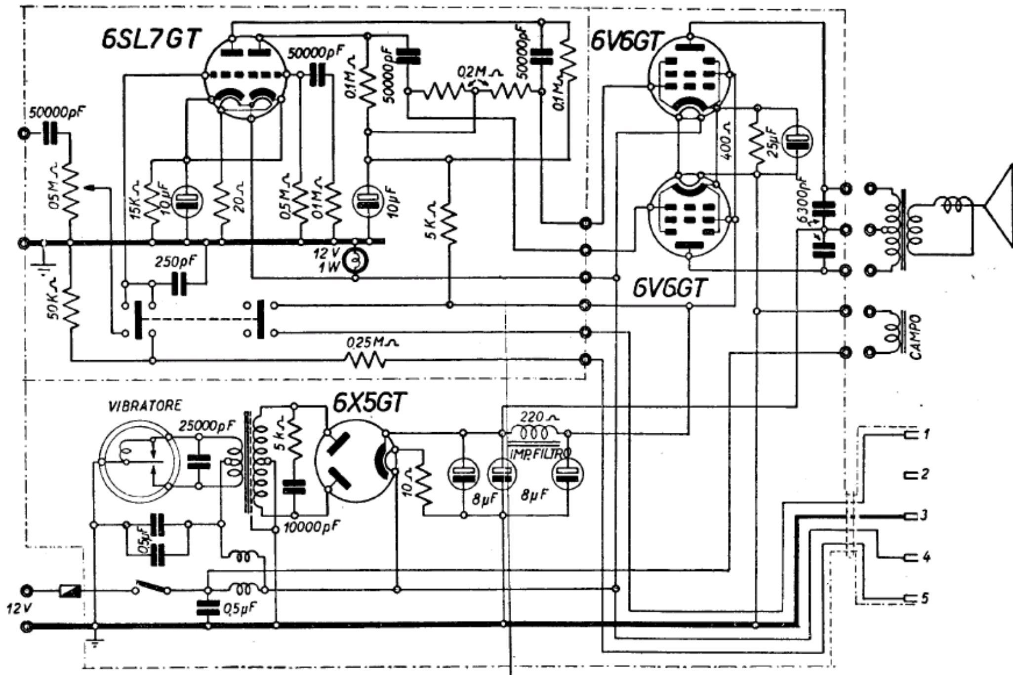
IRI « AUTOVOX » - Mod. RA 2/P - Complesso di amplificazione a bassa frequenza e di alimentazione a vibratore, per autopullmann.
